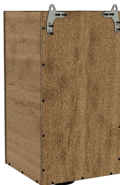
4. Assemblage des 2 pâtes de fixation sur la face arrière du réservoir avec 8 vis de 15 mm (trous pré-perçés)
