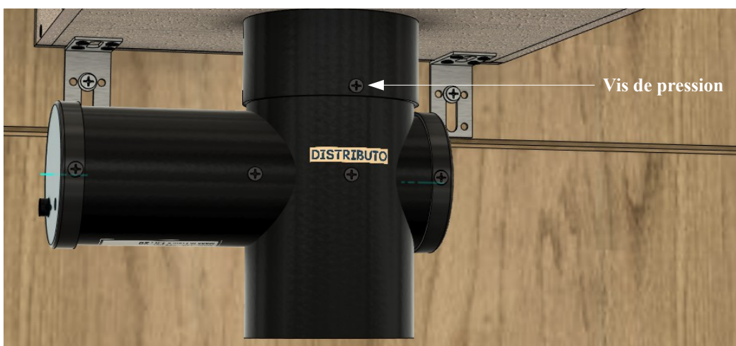
5. Emboîtement et blocage du doseur à l'aide de la vis de pression
